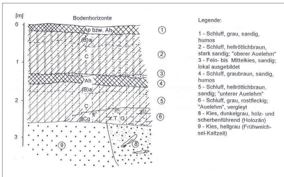
Abb. 5: „Normal-Profil“ der Pleißeau zwischen Zürcchau und Schmölln nach GLÄSSER (1995: 114).
